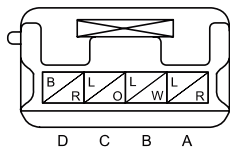
0915-102 天窗开关
