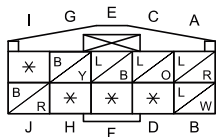
0915-101 天窗电机
