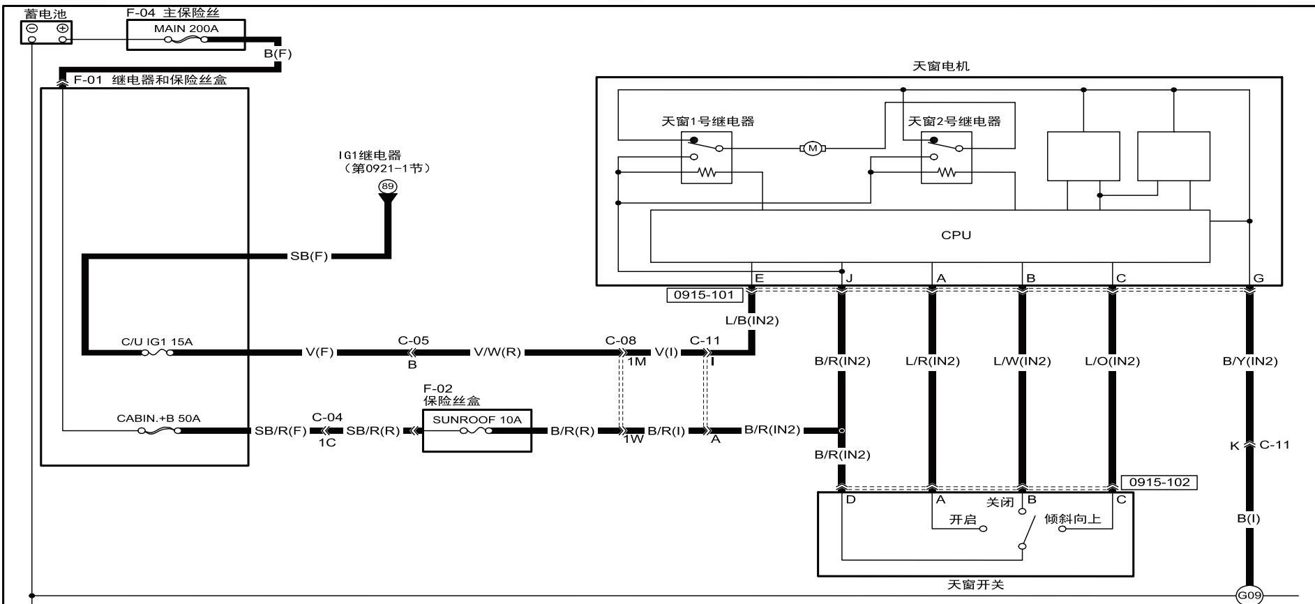
0915-101 天窗电机
